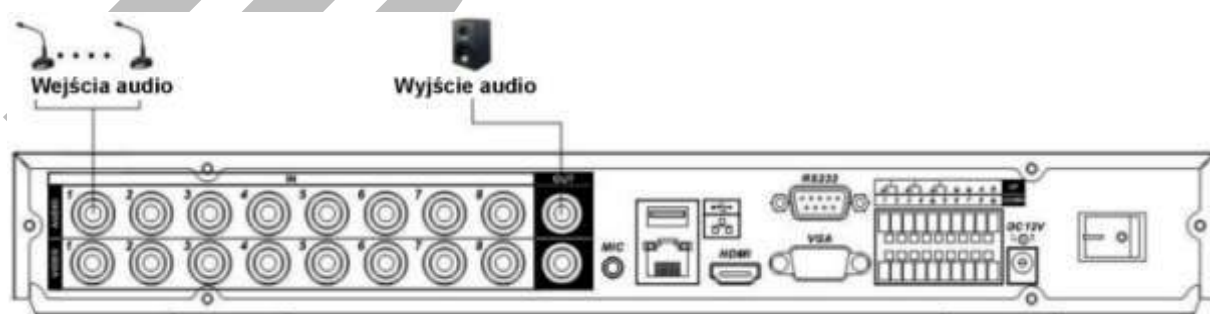
Rys. 3-3a. Podłączenia wejść i wyjść audio do rejestratora 8-kanalowego z serii LE-A.
