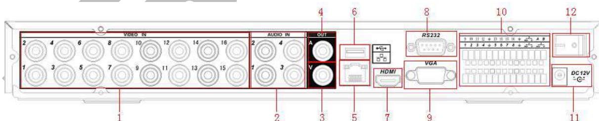
Rysunek 2-2c. Wygląd tylnego panelu rejestratora 16-kanałowego serii LE-A.
