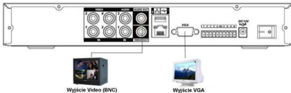
Rys. 3-2b Podłączenie monitorów do rejestratora LE-AS (LE-AN).
