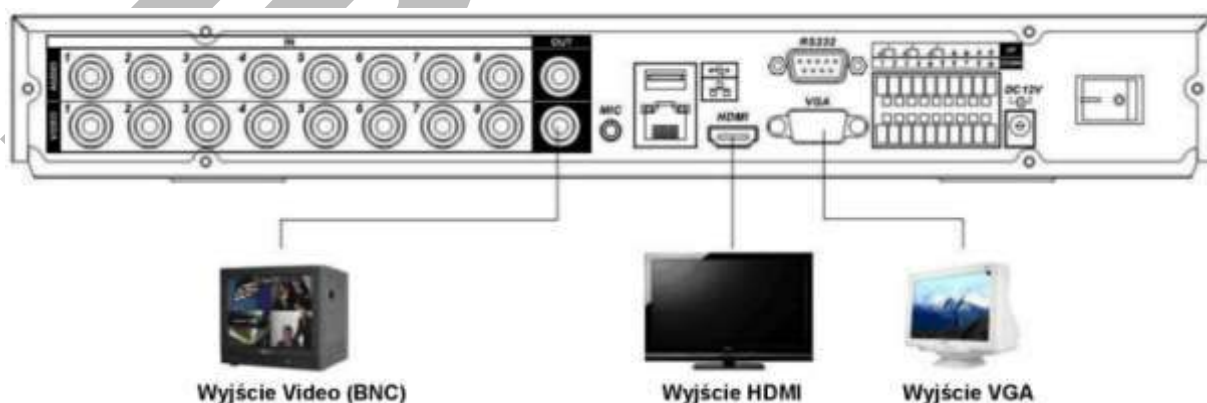
Rys. 3-2a. Podłączenie monitorów do rejestratora LE-A.
