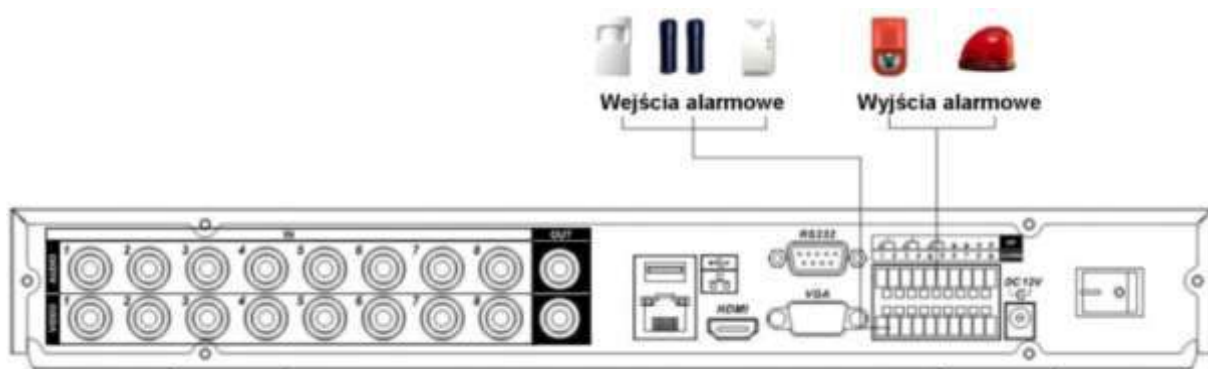
Rys. 3-4a. Podłączenie wejść i wyjść alarmowych w rejestratorach. serii LE-A.
