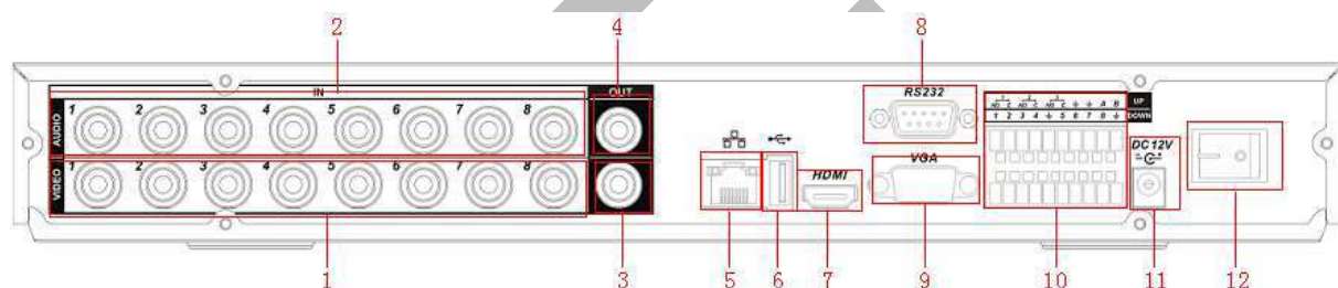
Rysunek 2-2b. Wygląd tylnego panelu rejestratora 8-kanałowego serii LE-A.
